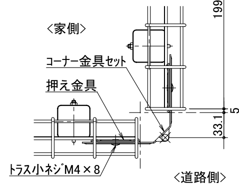
出隅コーナー納まり
