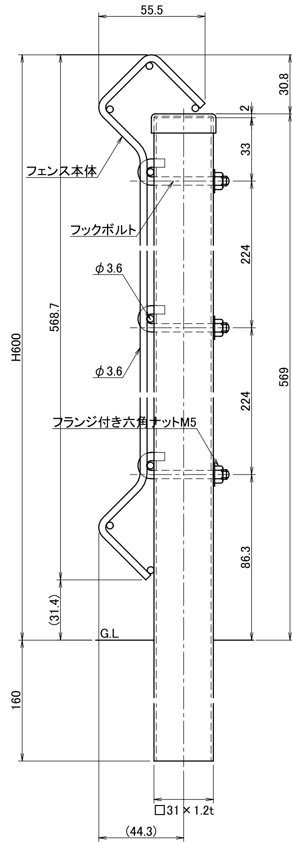
【側面図=1/2】
