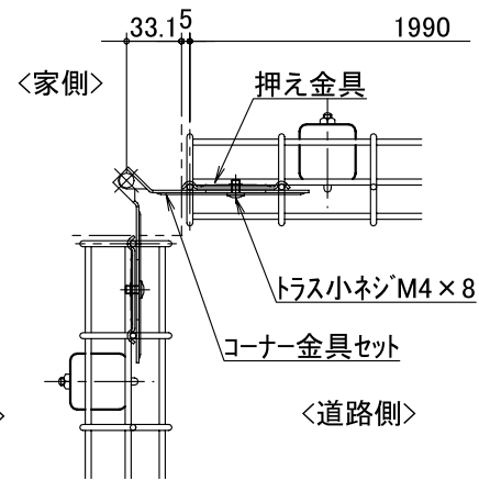
入隅コーナー納まり
