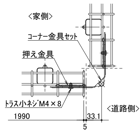
出隅コーナー納まり
