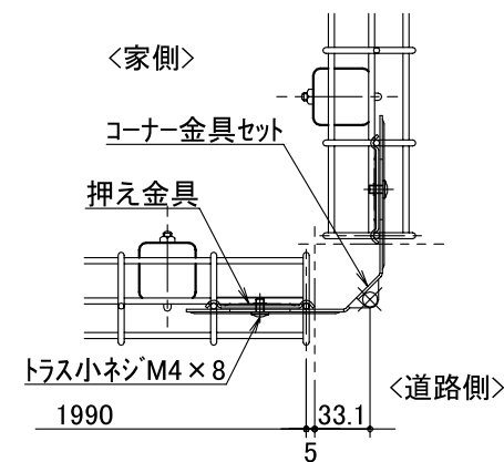
出隅コーナー納まり
