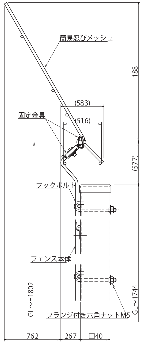
簡易忍び部詳細図 S=1/2
